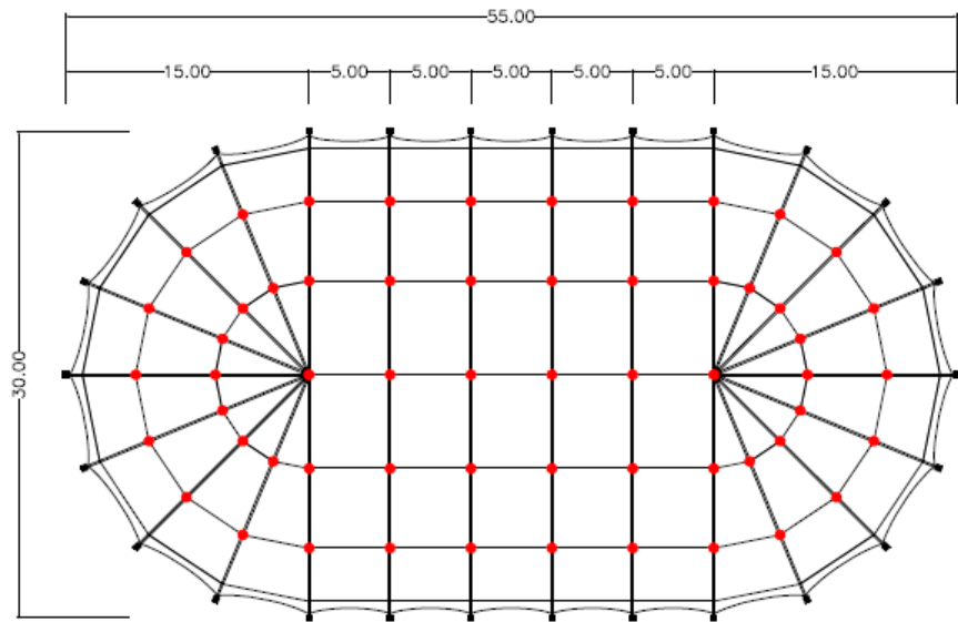
DRAUFSICHT
