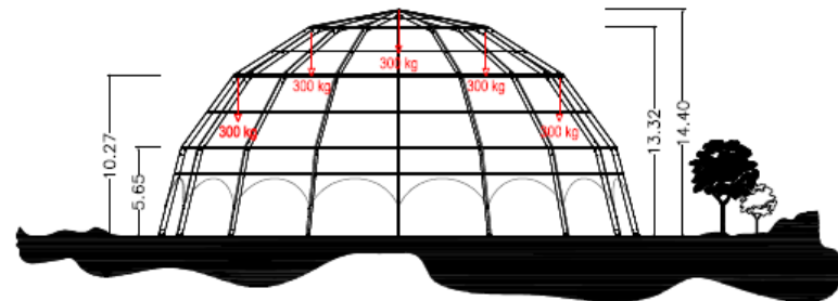
HAUPTANSICHT
