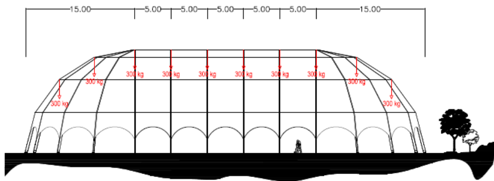
SEITENANSICHT
